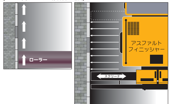
【ライン導水ブロック&縁石柵の場合】
