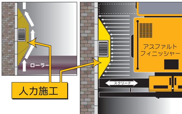
【通常の街渠柵の場合】
